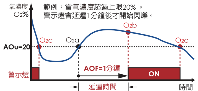
■ 氧濃度警報-警示燈延遲值(AOF)原理圖(選配)
