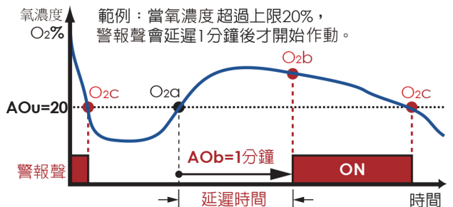
■ 氧濃度警報-警報聲延遲值(AOb)原理圖(選配)
