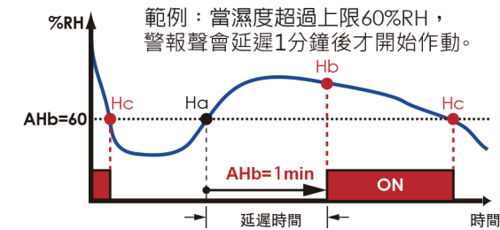
■ 濕度警報聲動作延遲值(AHb)原理圖
