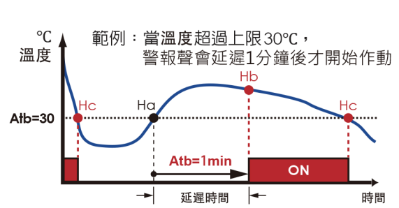
■ 溫度警報聲動作延遲值(Atb)原理圖
