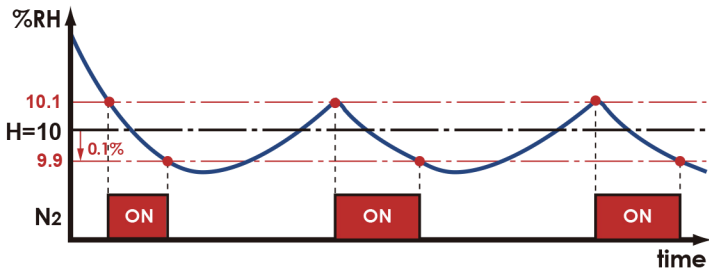
■ 濕度設定動作原理圖
