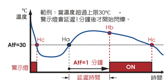
■ 溫度警報-警示燈延遲值(AtF)原理圖
