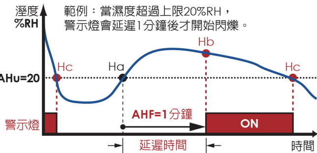
■ 濕度警報-警示燈延遲值(AHF)原理圖
